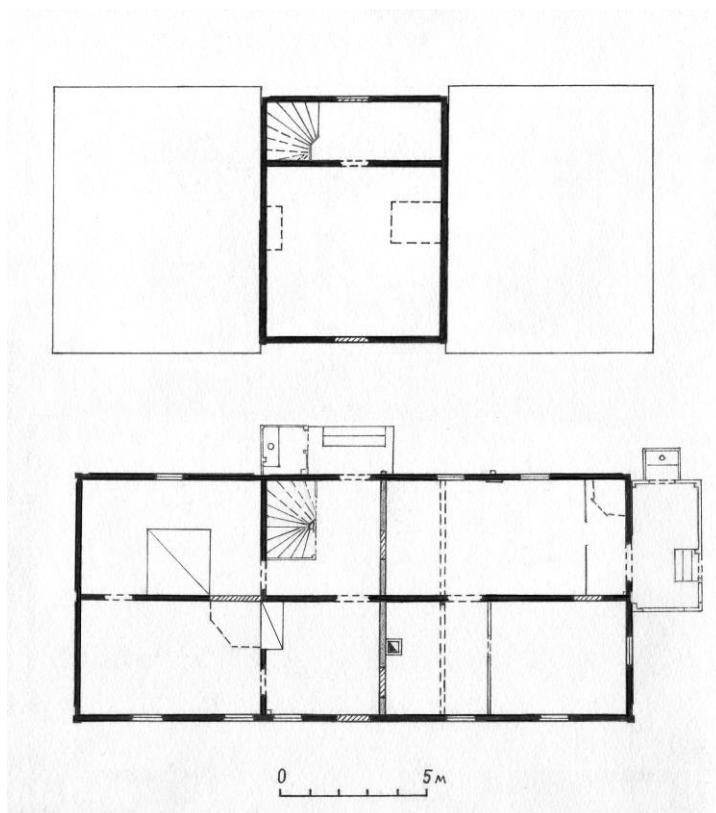
Ил. 9. Дом в Опанаскове. Поэтажные планы на 1993 г. Прерывистой чертой показаны разобранные печи и перемещенная капитальная стена
