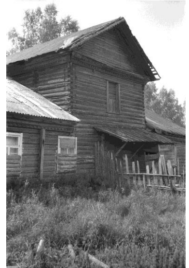
Ил. 3. Мезонин с прорезными причелинами, обломками ригеля-схватки и следами исчезнувшего балкона с двухскатной кровлей. Фото 1993 г.
